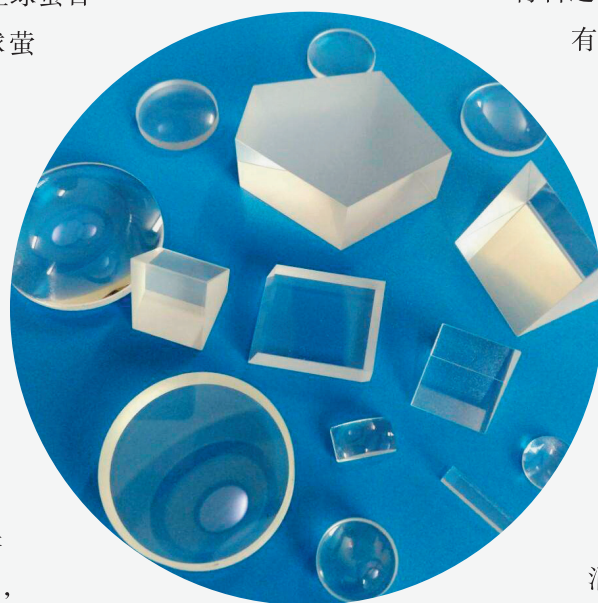
＞ 萤石用作光学棱镜（图片来自网络）
